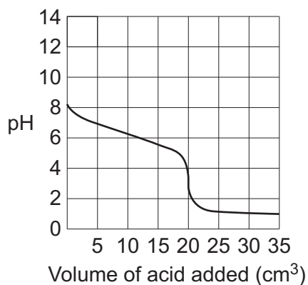
Titration curve
